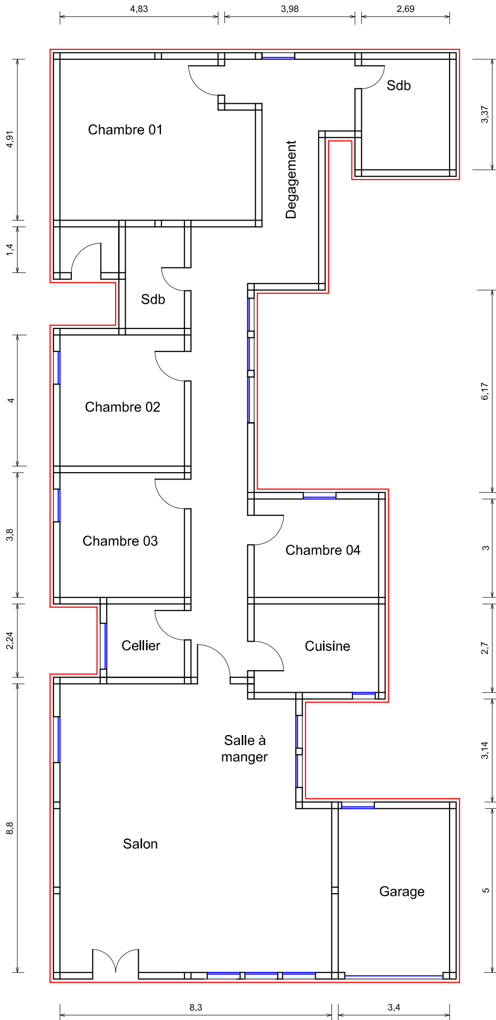
PLAN : Modifié
